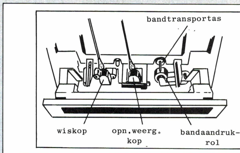
Fig. 2. Een goede opname is niet mogelijk met vervuilde koppen! Maak koppen, bandtransportas en bandaandrukrol steeds regelmatig schoon, dat wil zeggen steeds na 15 à 20 spelluren.
