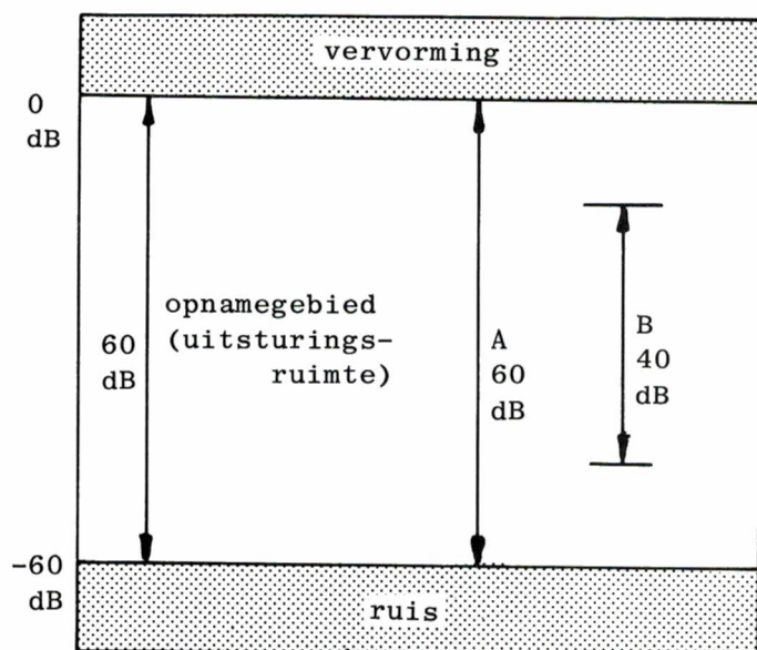
Fig. 1. De opname speelt zich af in het gebied tussen vervorming (maximale uitsturing) en ruis (minimale uitsturing).
