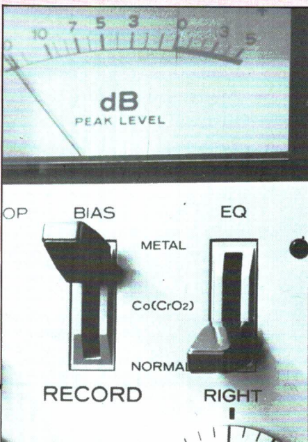
Foto 4. De bias- en Eq-schakelaar kunnen best wel eens in een afwijkende stand worden geplaatst. En ook kan het soms wel eens nuttig zijn het ruisonderdrukkingssysteem (NR-system) uitgeschakeld te laten.
